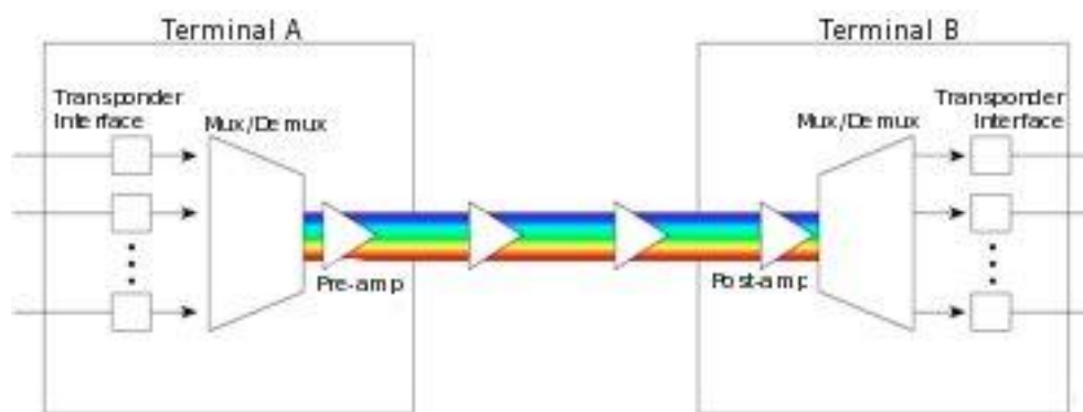
Gambar 1. Konfigurasi Perangkat Coarse-Wavelength Digital Multiplexer (CWDM)
